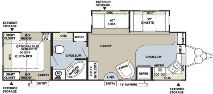
829RKSS 32'2" - 9,80m
