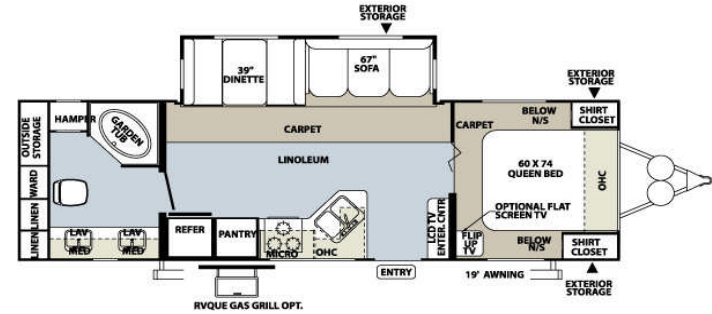
829RGSS 32'2" - 9,80m
