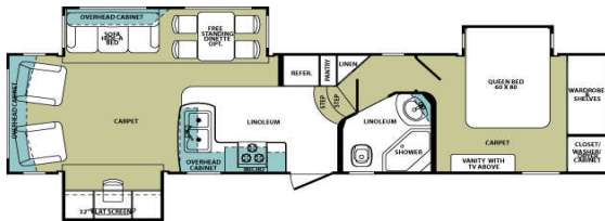
3150 RL 37' 5" (11.4 m)
